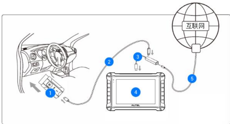
图 18-1 “远程专家”技师端连接示意图
